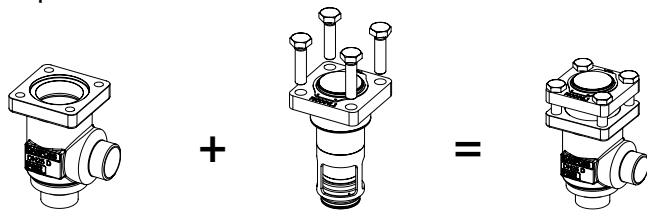
Корпус клапана, размер 25 (1"), сварка встык DIN, угловой, 148B5452
