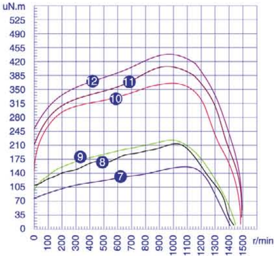
Torque(50Hz)
